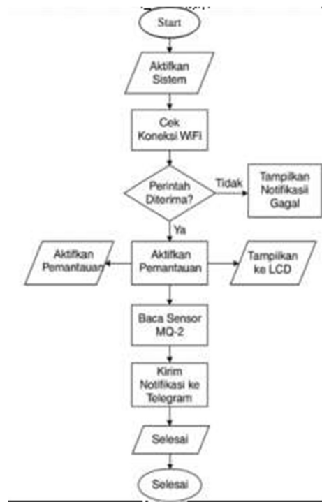
Gambar 9. Alur Sistem Kerja Sistem Otomatis Kualitas Udara
